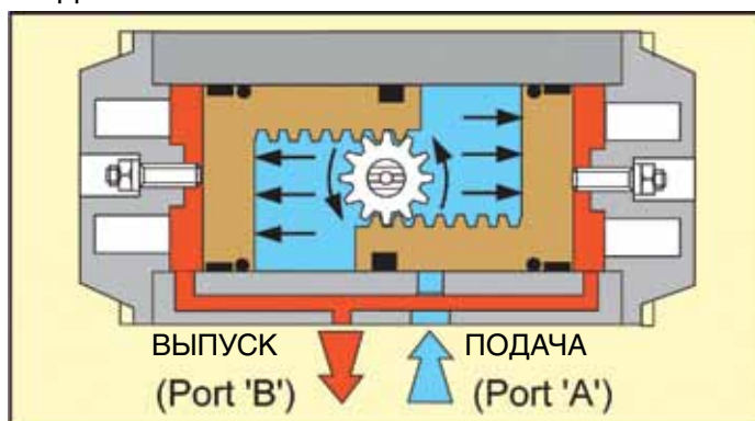
ДВИЖЕНИЕ ПОРШНЕЙ ПРИ ОТКРЫВАНИИ
